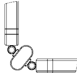
Aufbauvariante mit einfachem Beschlagsatz
